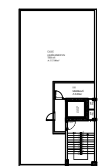
ÇATI KATI PLANI A:185.00 M2
