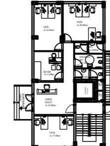
ZEMİN KAT PLANI A:145.00 M2
