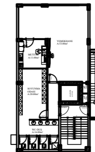
BODRUM KAT PLANI A:145.00 M2
